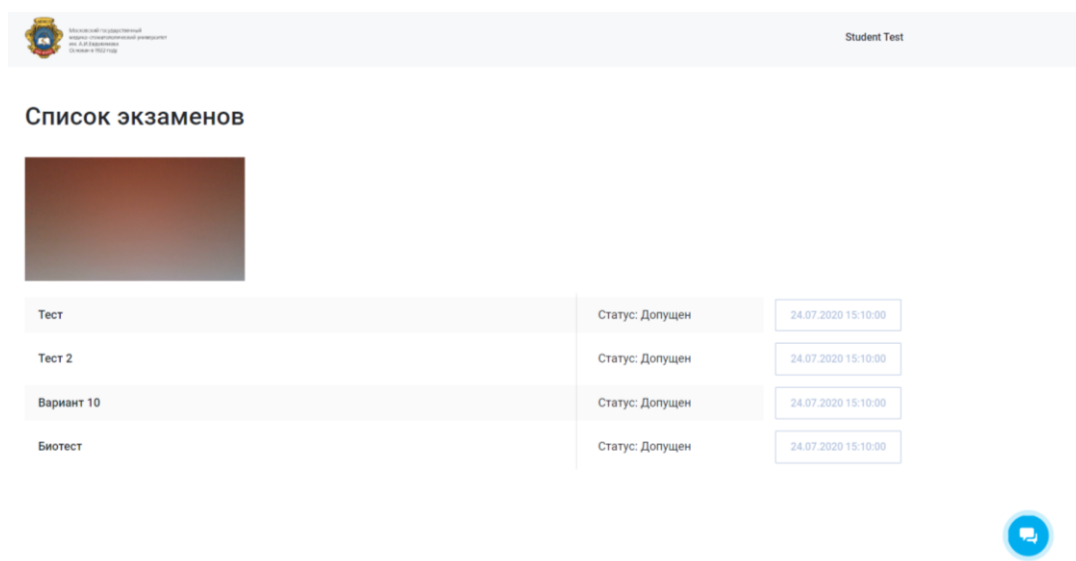
Рисунок 4. Список экзаменов.
