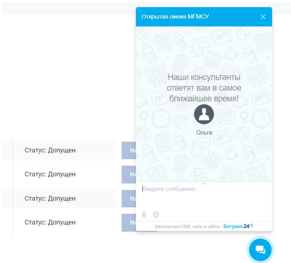
Рисунок 5. Чат.
